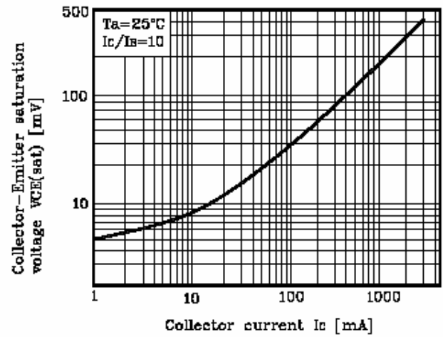
Fig. 2 V_{CE(sat)} - I_C
