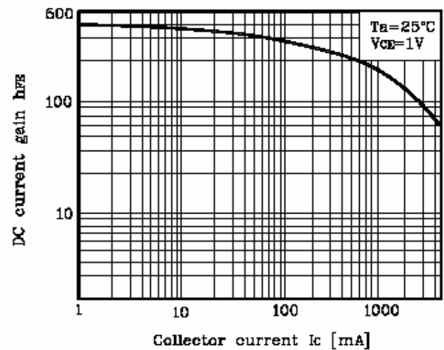
Fig. 4 h_{FE} - I_C
